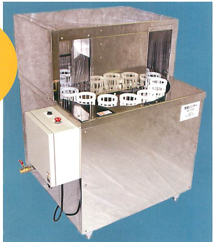
↑簡易リンサーMR-1000 16バスケット、正逆回転可、インバーター付き
