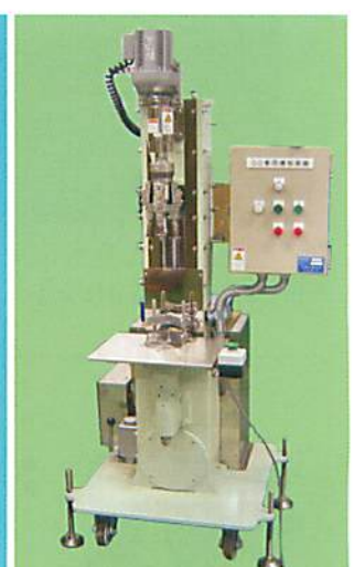
↑SO型半自動 PPキャップ
